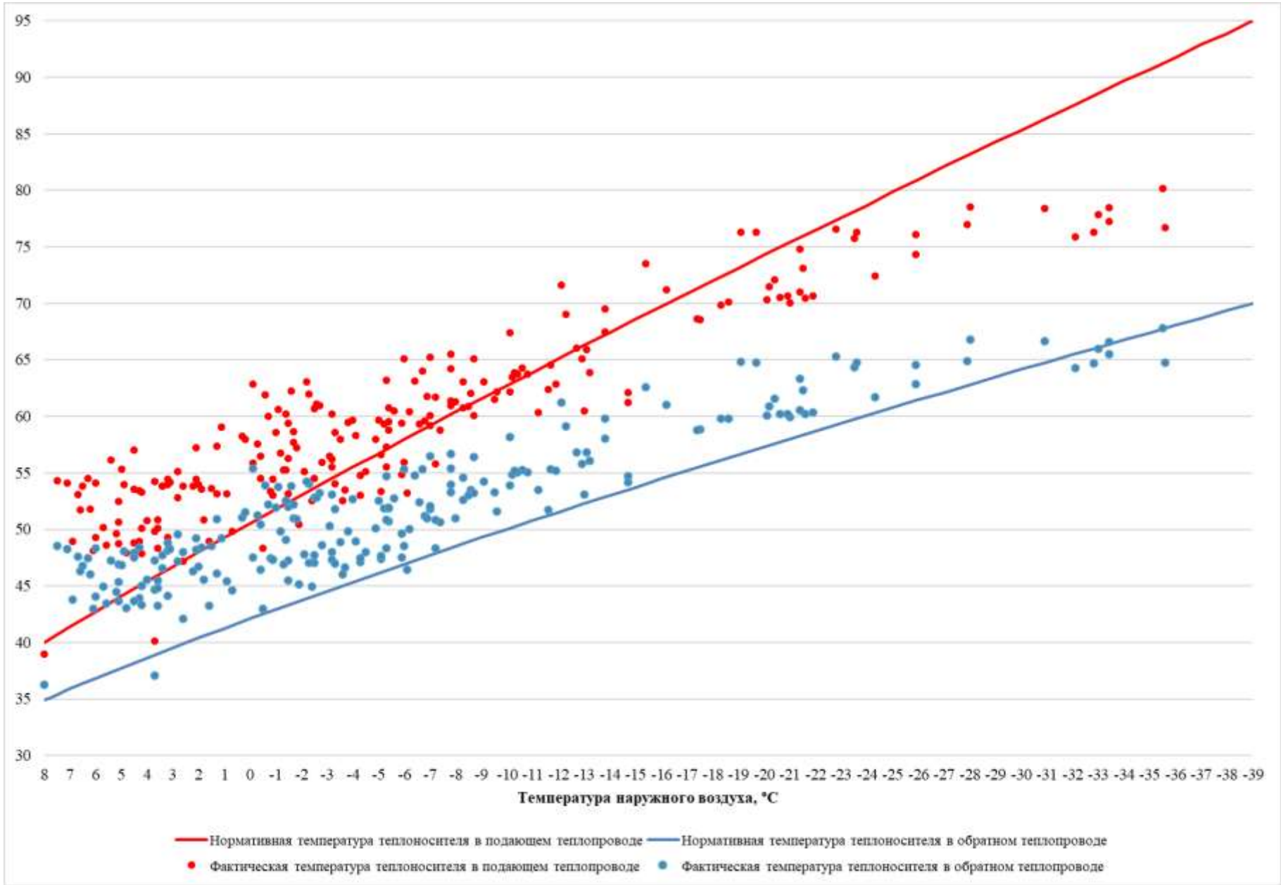
Рисунок 3.33 – Сравнение утвержденного и фактического температурных графиков за 2023 г. – Котельная №2 п. Разъезд-Абагуровский
