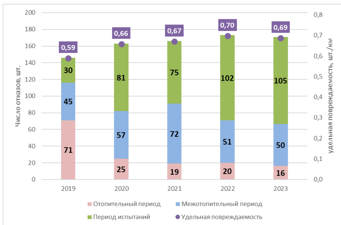
Рисунок 3.47 – Повреждаемость магистральных тепловых сетей
