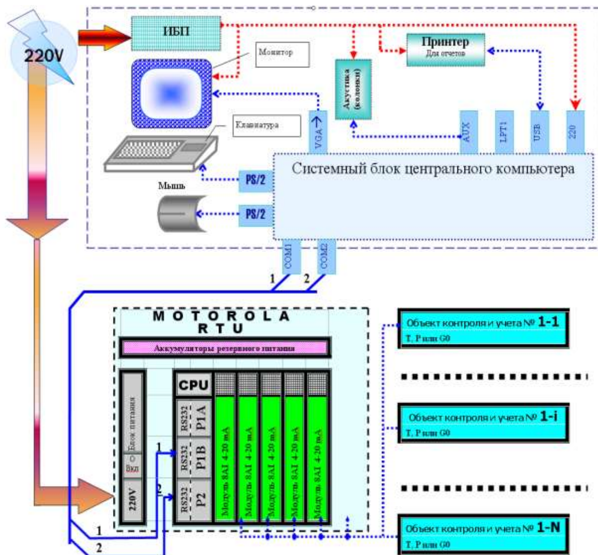
Рисунок 2.6 – Структурная схема информационно-измерительного комплекса
