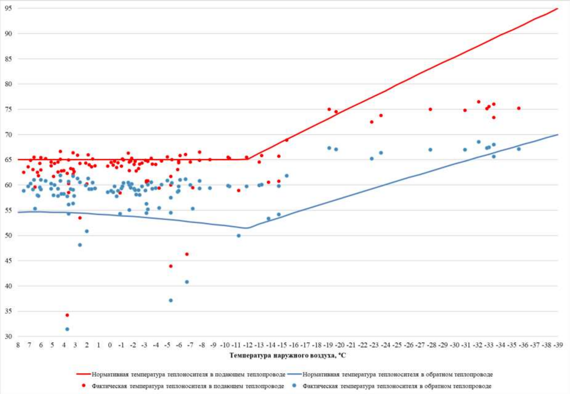
Рисунок 3.36 – Сравнение утвержденного и фактического температурных графиков за 2023 г. – Котельная ОЦ «Голубь»
