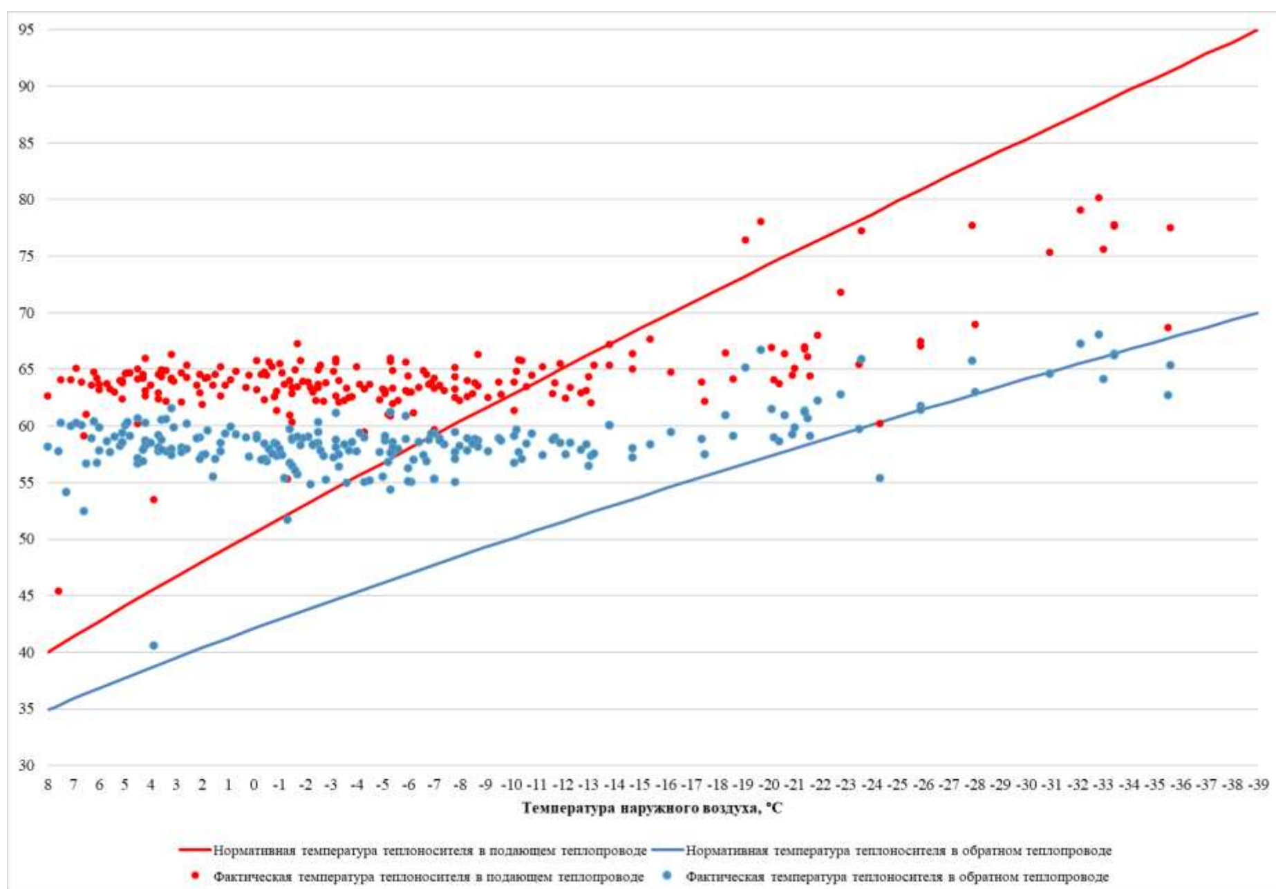
Рисунок 3.44 – Сравнение утвержденного и фактического температурных графиков за 2023 г. – Котельная ст. Полосухино
