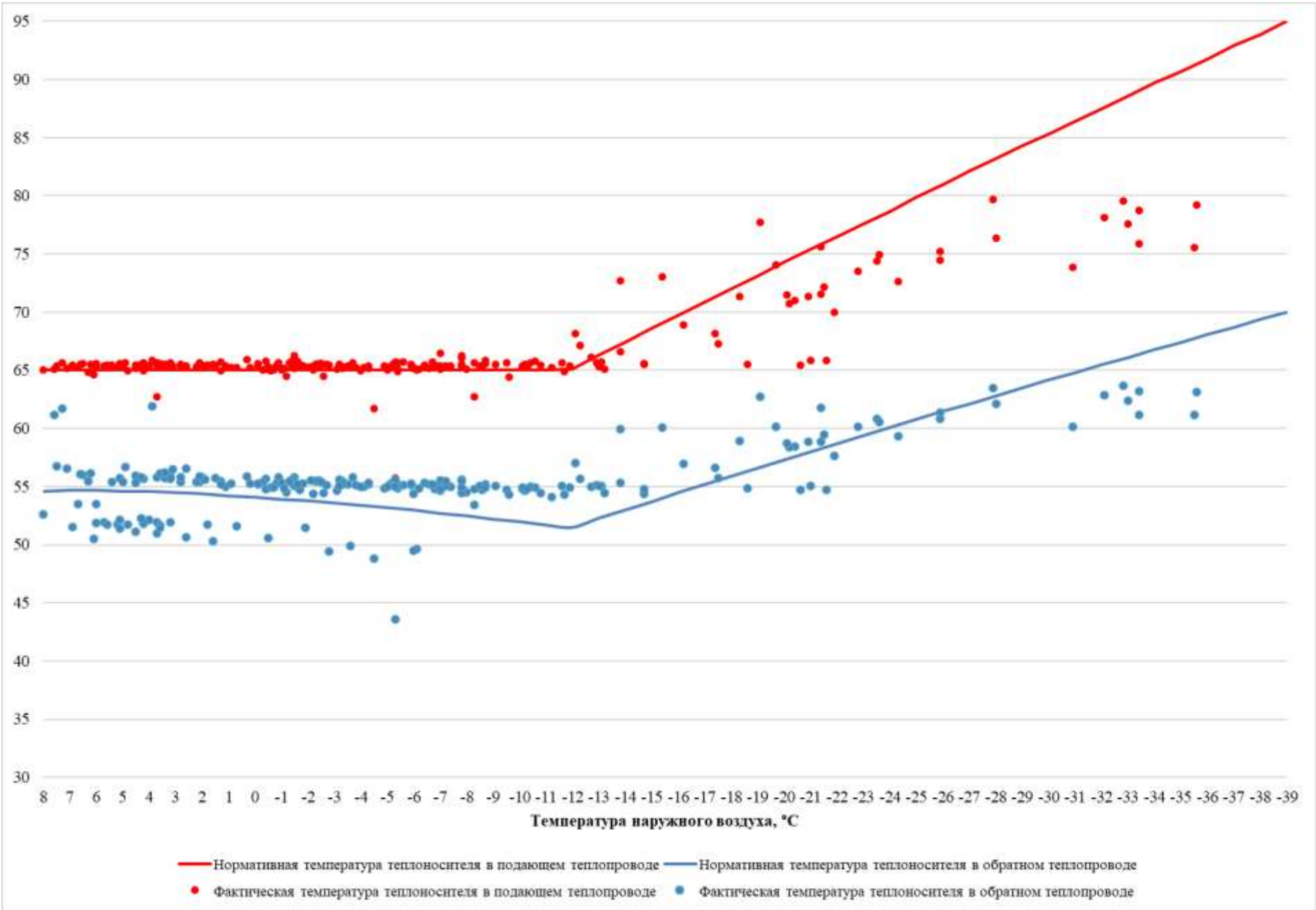
Рисунок 3.19 – Сравнение утвержденного и фактического температурных графиков за 2023 г. – Зырянская районная котельная
