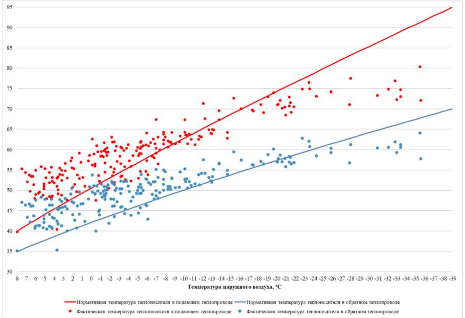
Рисунок 3.32 – Сравнение утвержденного и фактического температурных графиков за 2023 г. – Котельная №1 п. Разъезд-Абагуровский
