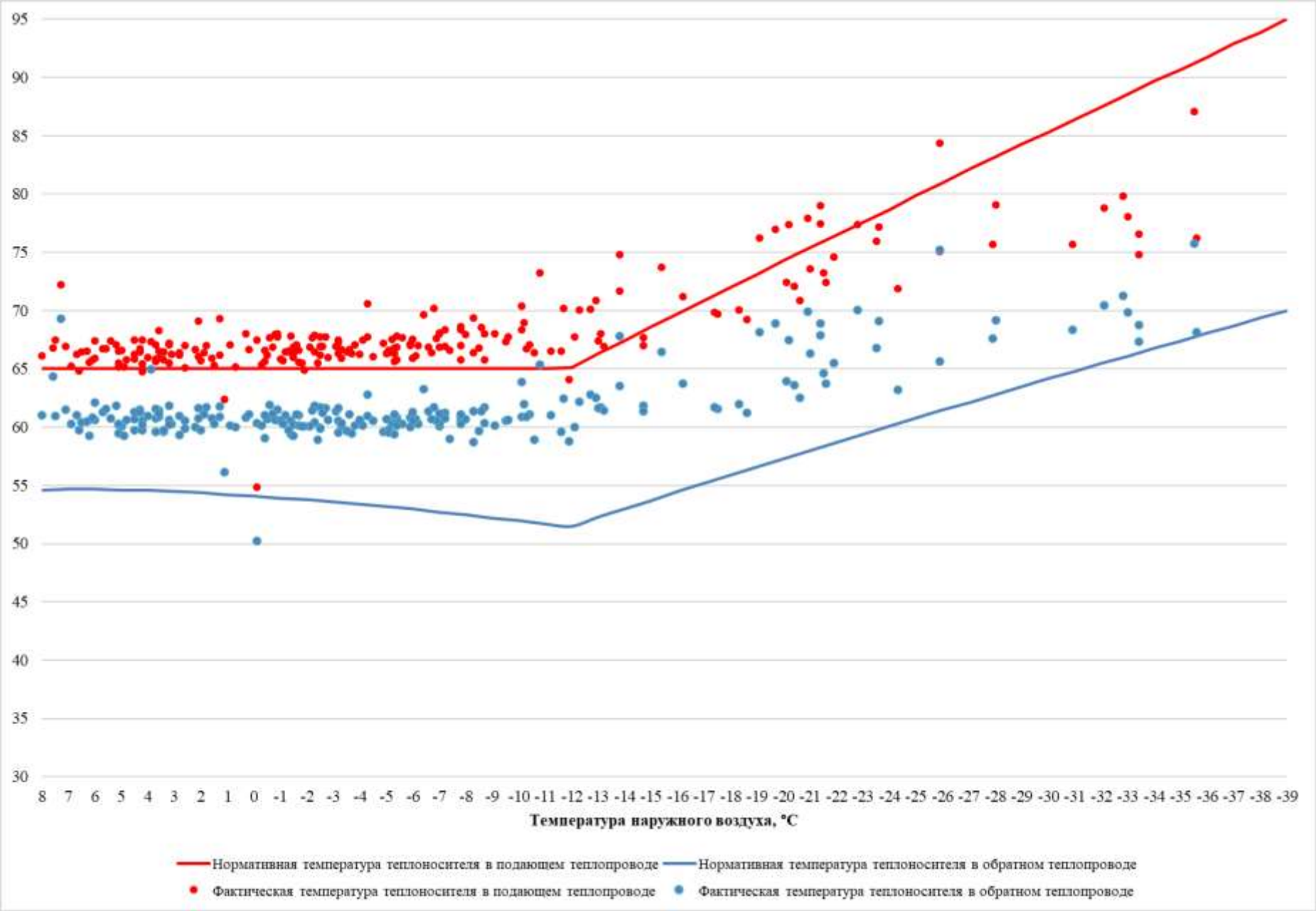
Рисунок 3.35 – Сравнение утвержденного и фактического температурных графиков за 2023 г. – Котельная «РТРС»
