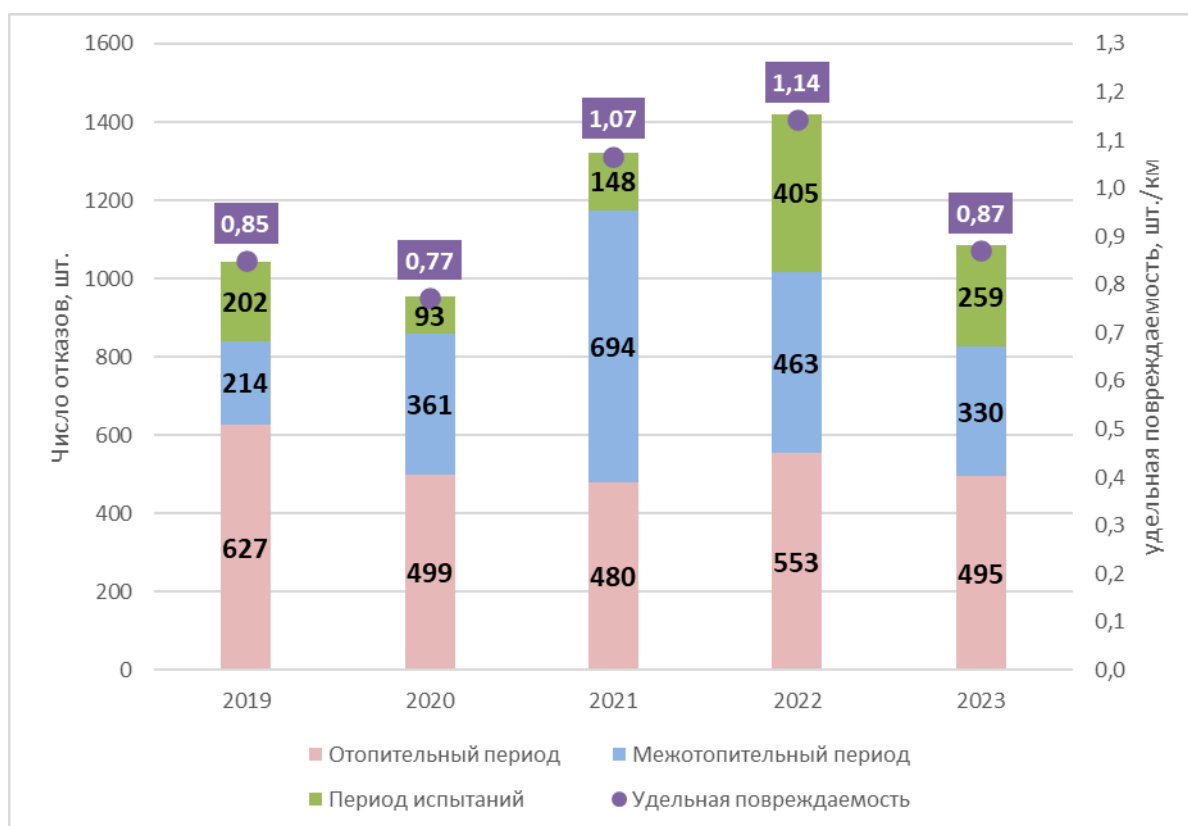
Рисунок 3.48 – Повреждаемость распределительных тепловых сетей и сетей ГВС
