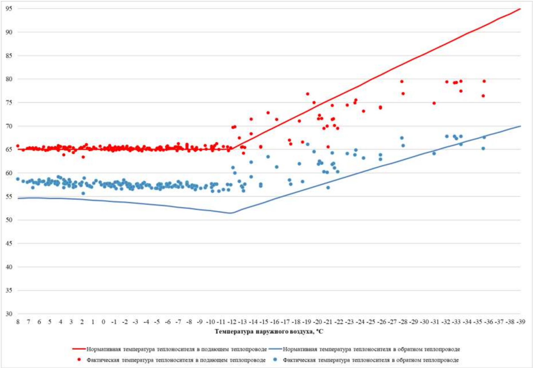
Рисунок 3.29 – Сравнение утвержденного и фактического температурных графиков за 2023 г. – Котельная пос. Листвяги
