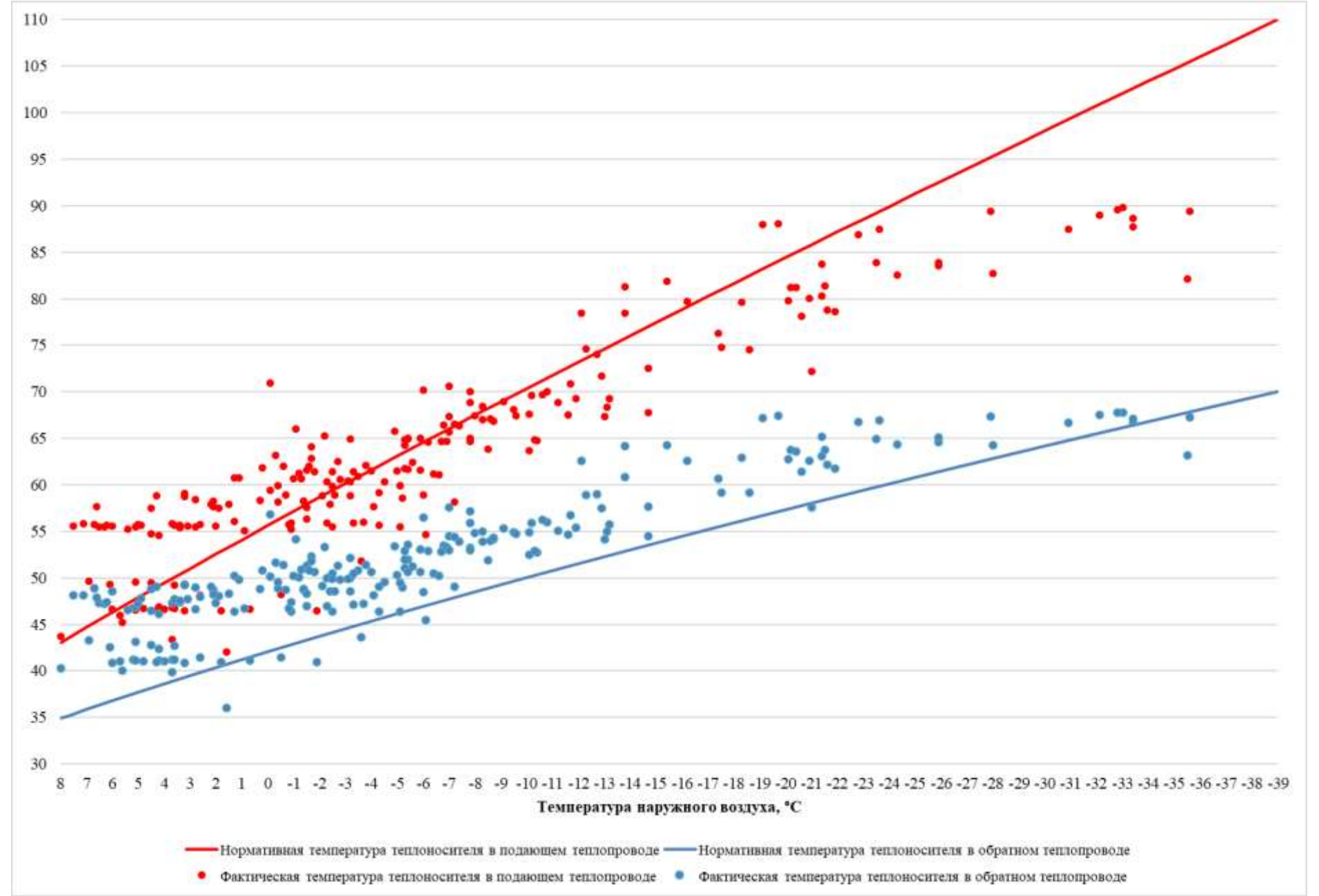
Рисунок 3.20 – Сравнение утвержденного и фактического температурных графиков за 2023 г. – Куйбышевская центральная котельная
