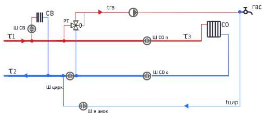
Рисунок 3.53 – Потребитель с открытым водоразбором на ГВС и непосредственным присоединением СО
