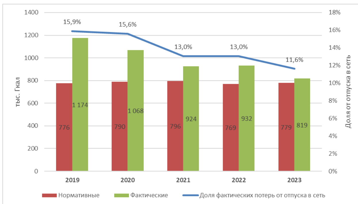
Рисунок 3.51 – Сравнение нормативных и фактических потерь тепловой энергии в тепловых сетях
