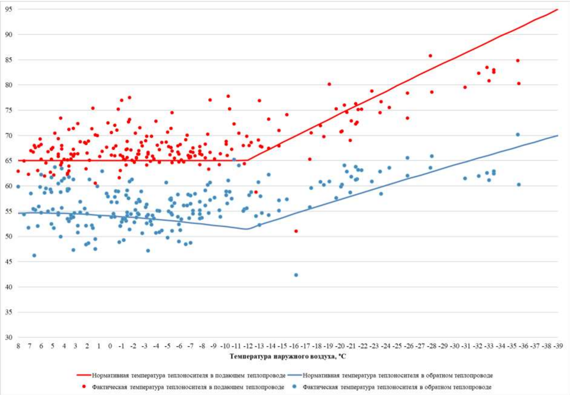
Рисунок 3.23 – Сравнение утвержденного и фактического температурных графиков за 2023 г. – Котельная №72
