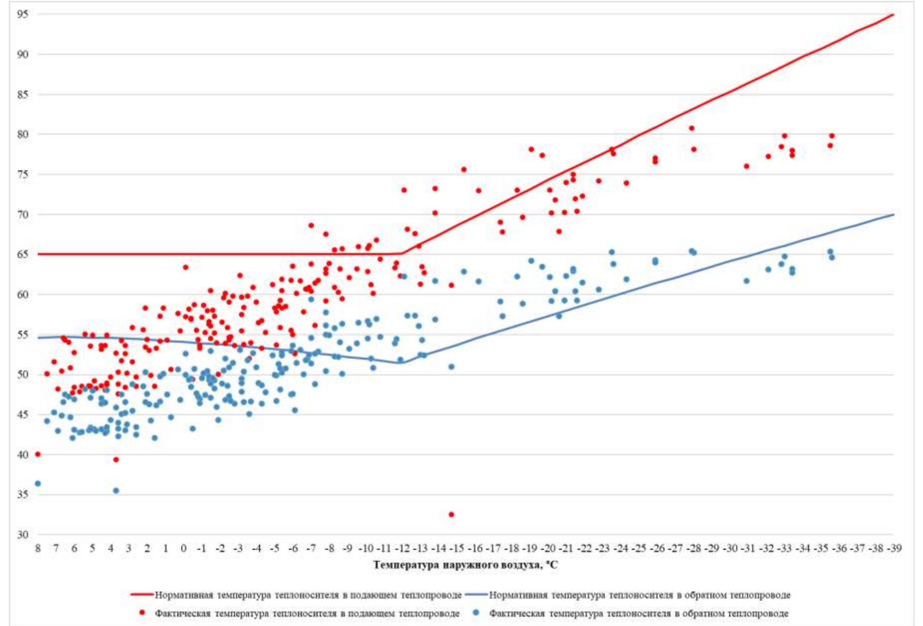
Рисунок 3.26 – Сравнение утвержденного и фактического температурных графиков за 2023 г. – Котельная №1 п. Абагур-Лесной
