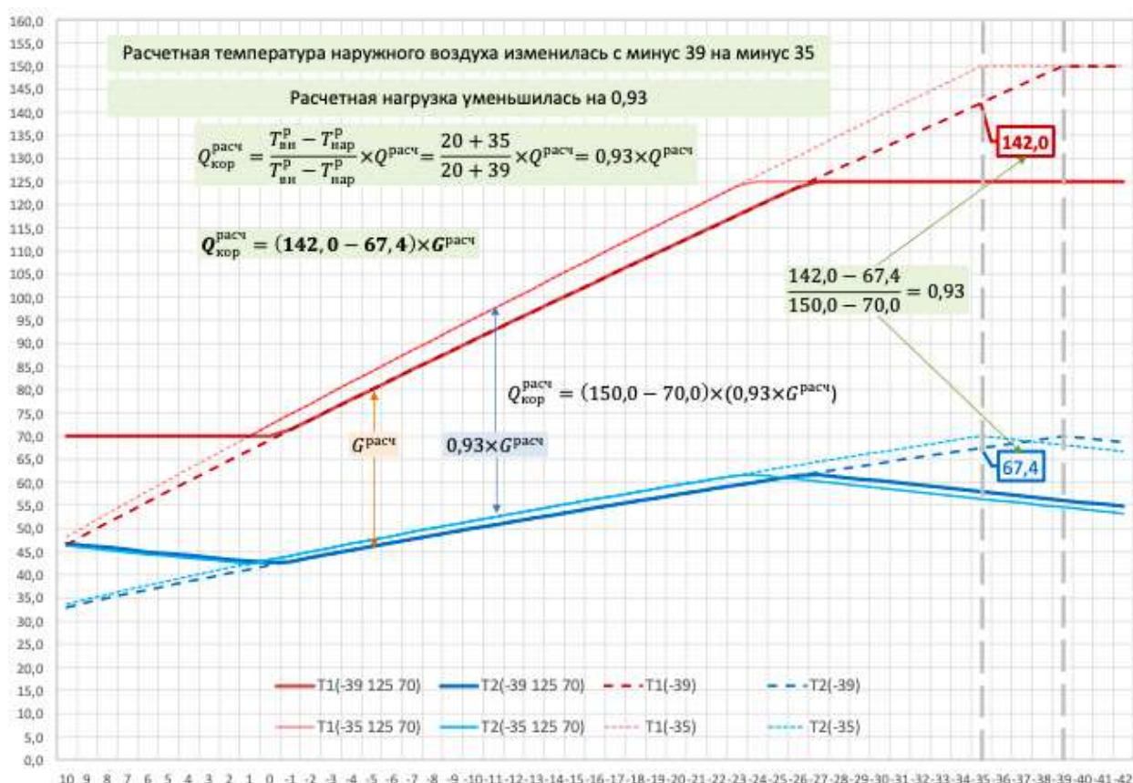
Рисунок 3.10 – Варианты пересмотра температурного графика при повышении расчетной температуры наружного воздуха: с сохранением и с уменьшением расхода сетевой воды
