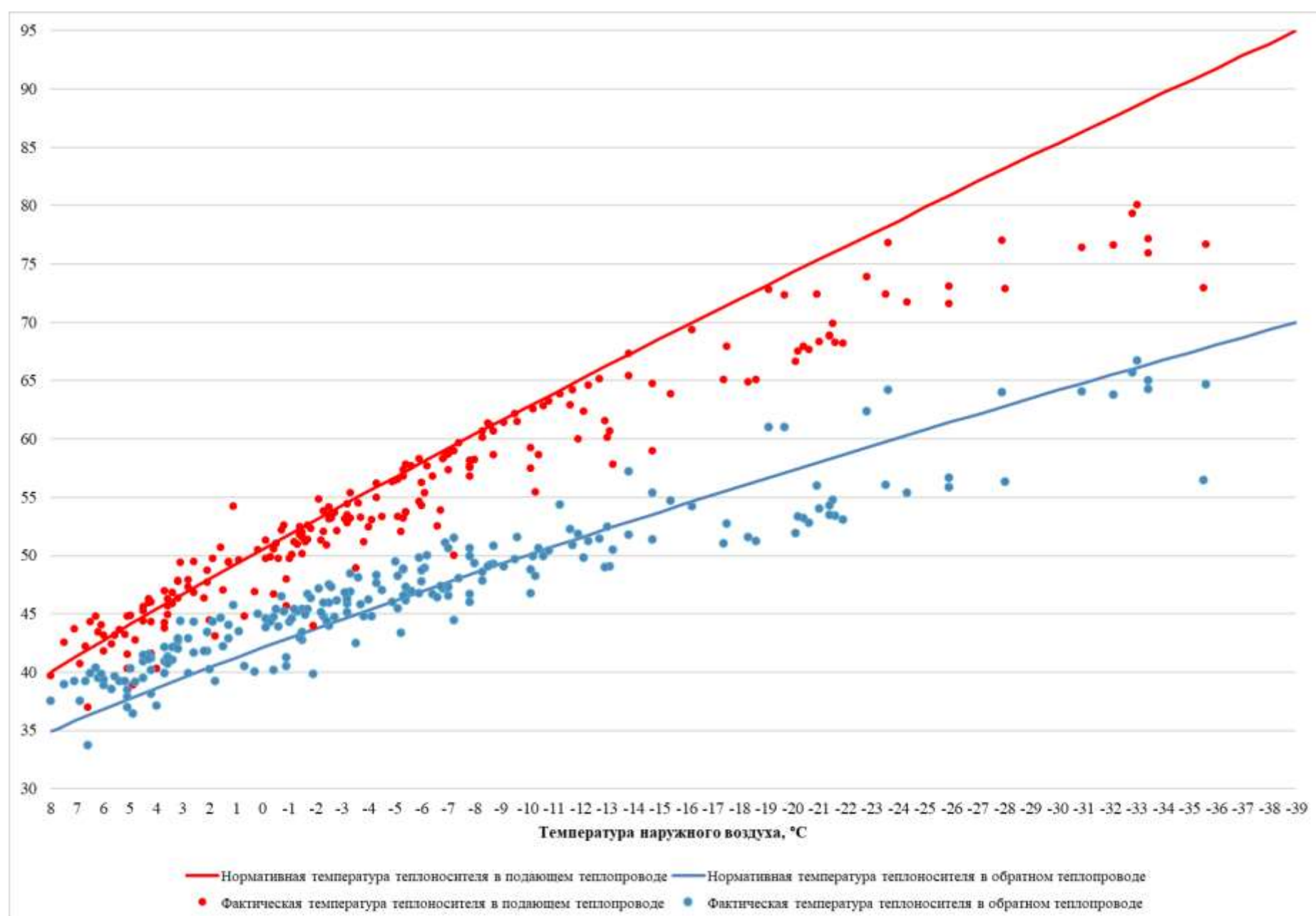
Рисунок 3.43 – Сравнение утвержденного и фактического температурных графиков за 2023 г. – Котельная детского сада №123
