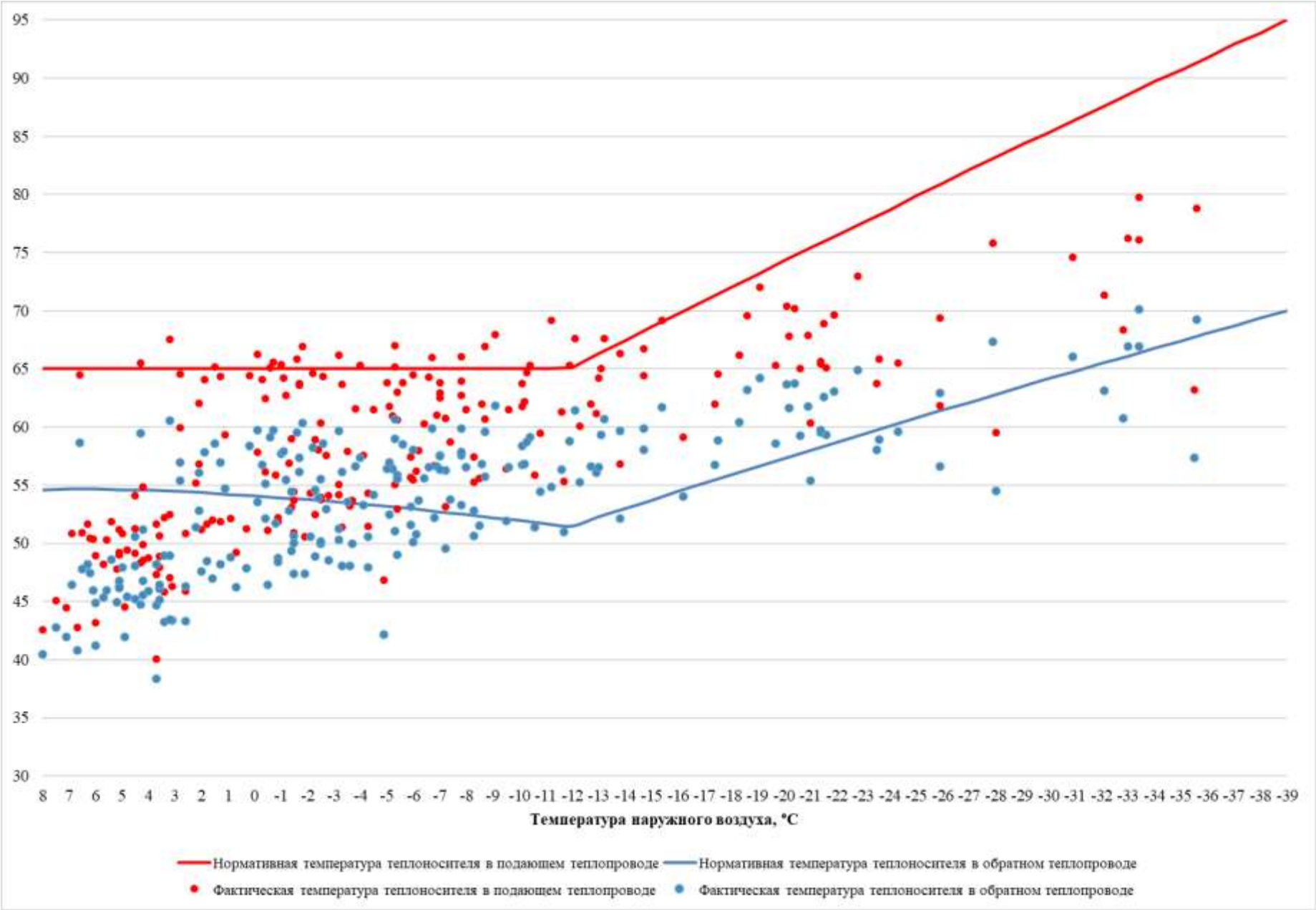
Рисунок 3.40 – Сравнение утвержденного и фактического температурных графиков за 2023 г. – Котельная школы №43
