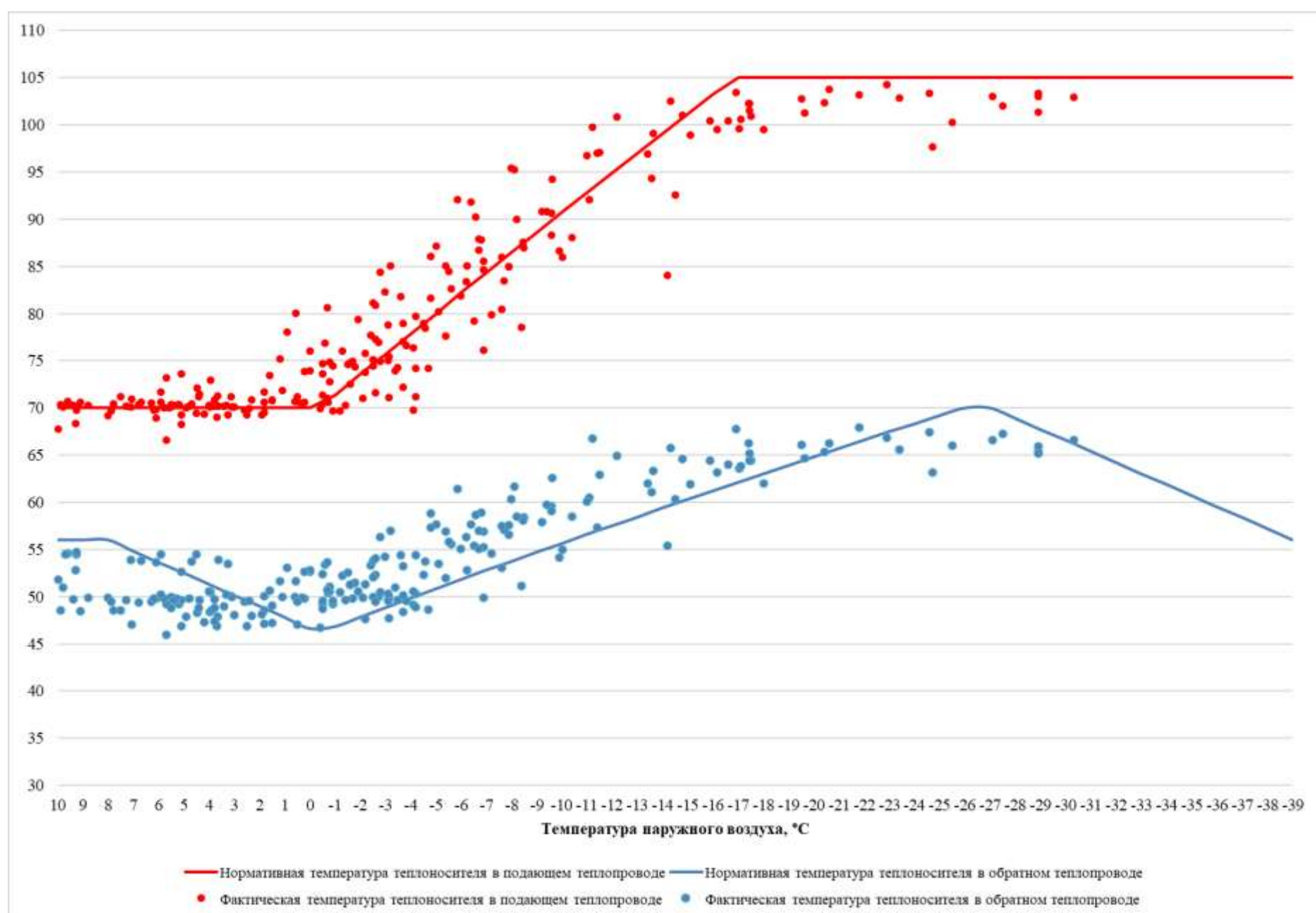
Рисунок 3.15 – Сравнение утвержденного и фактического температурных графиков за 2023 г. – Новоильинская газовая котельная
