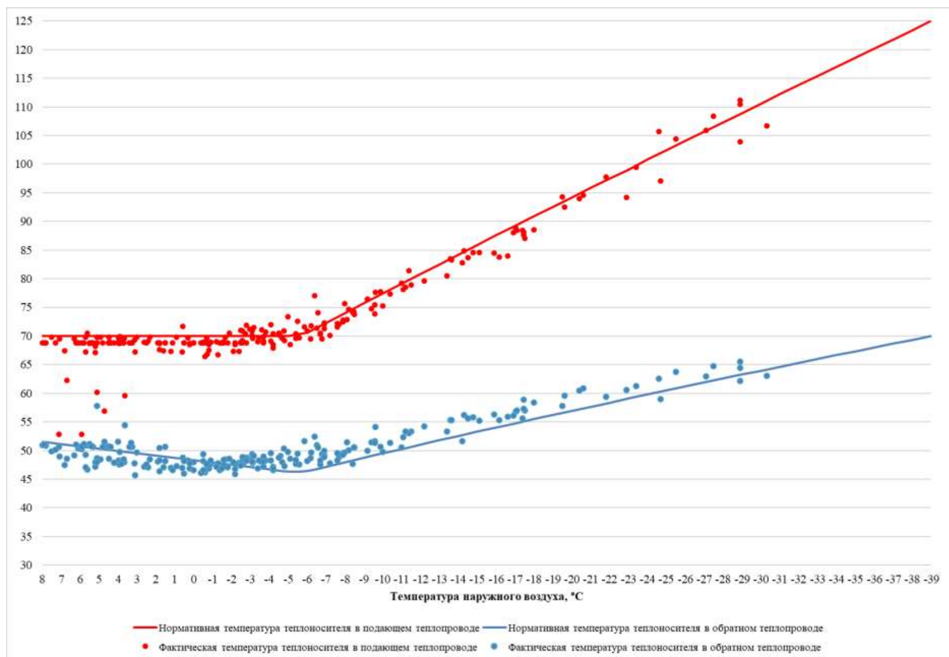
Рисунок 3.16 – Сравнение утвержденного и фактического температурных графиков за 2023 г. – Котельная кв. 24
