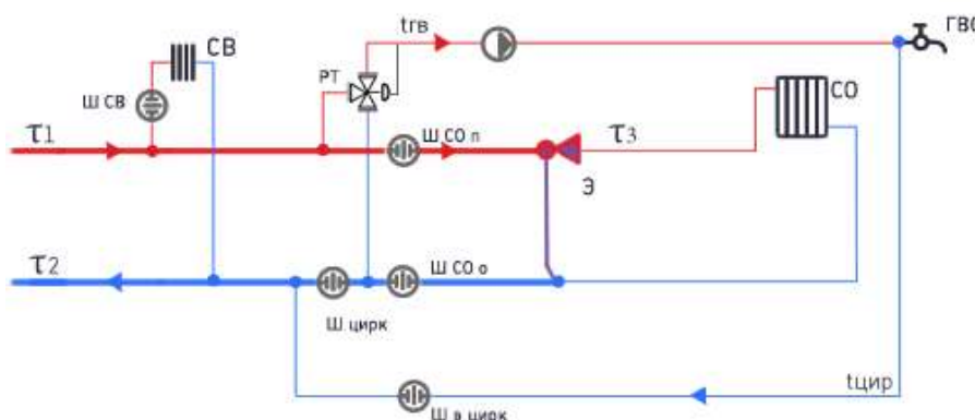
Рисунок 3.52 – Потребитель с открытым водоразбором на ГВС и элеваторным присоединением систем отопления (СО)
