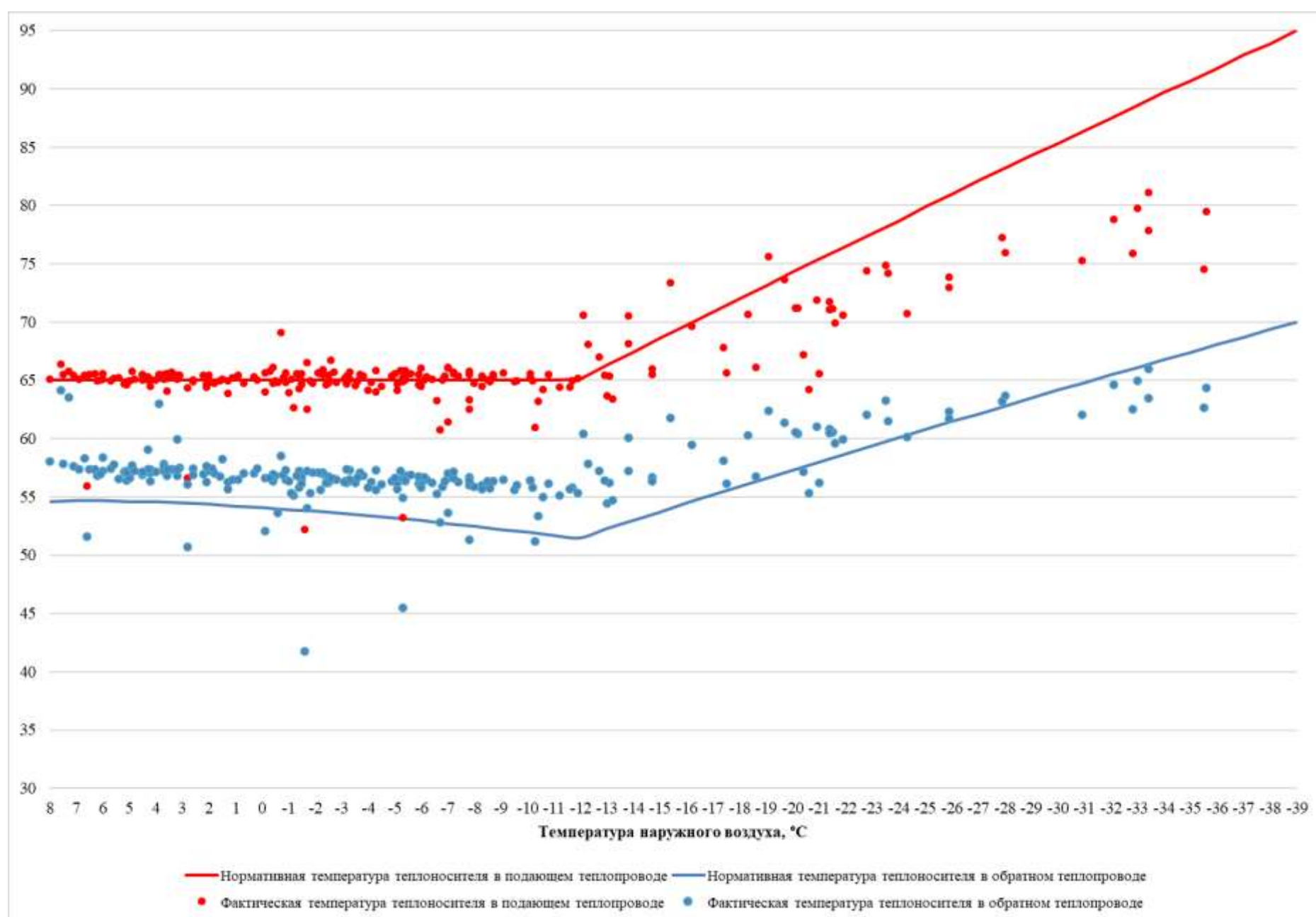
Рисунок 3.18 – Сравнение утвержденного и фактического температурных графиков за 2023 г. – Байдаевская центральная котельная №2
