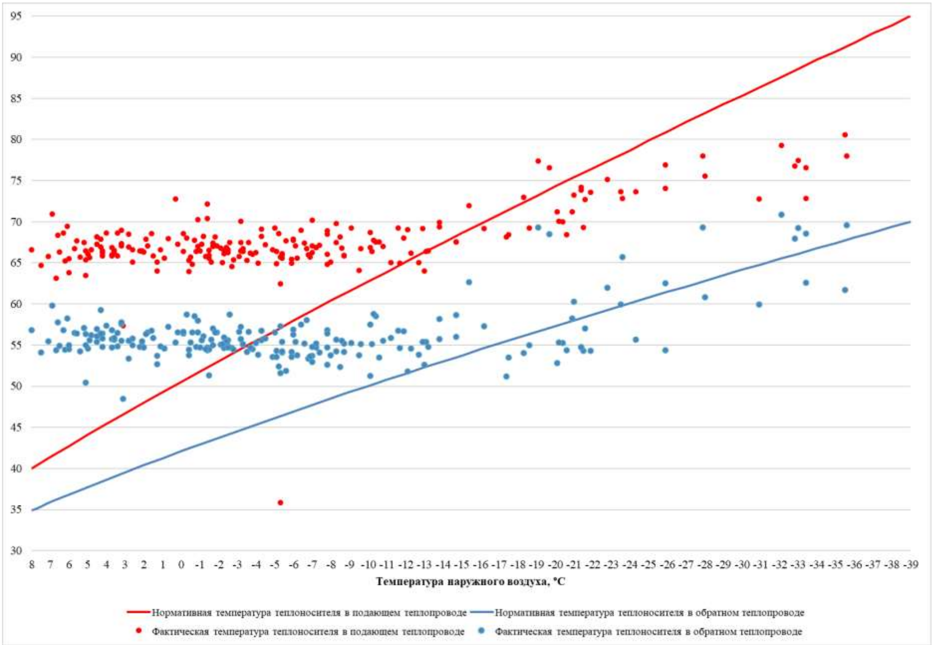
Рисунок 3.34 – Сравнение утвержденного и фактического температурных графиков за 2023 г. – Котельная проф. «Бунгурский»
