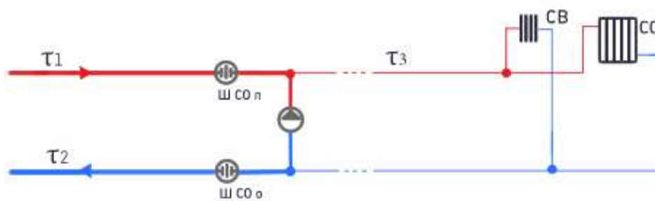
Рисунок 3.8 – ЦТП с насосным присоединением СО
