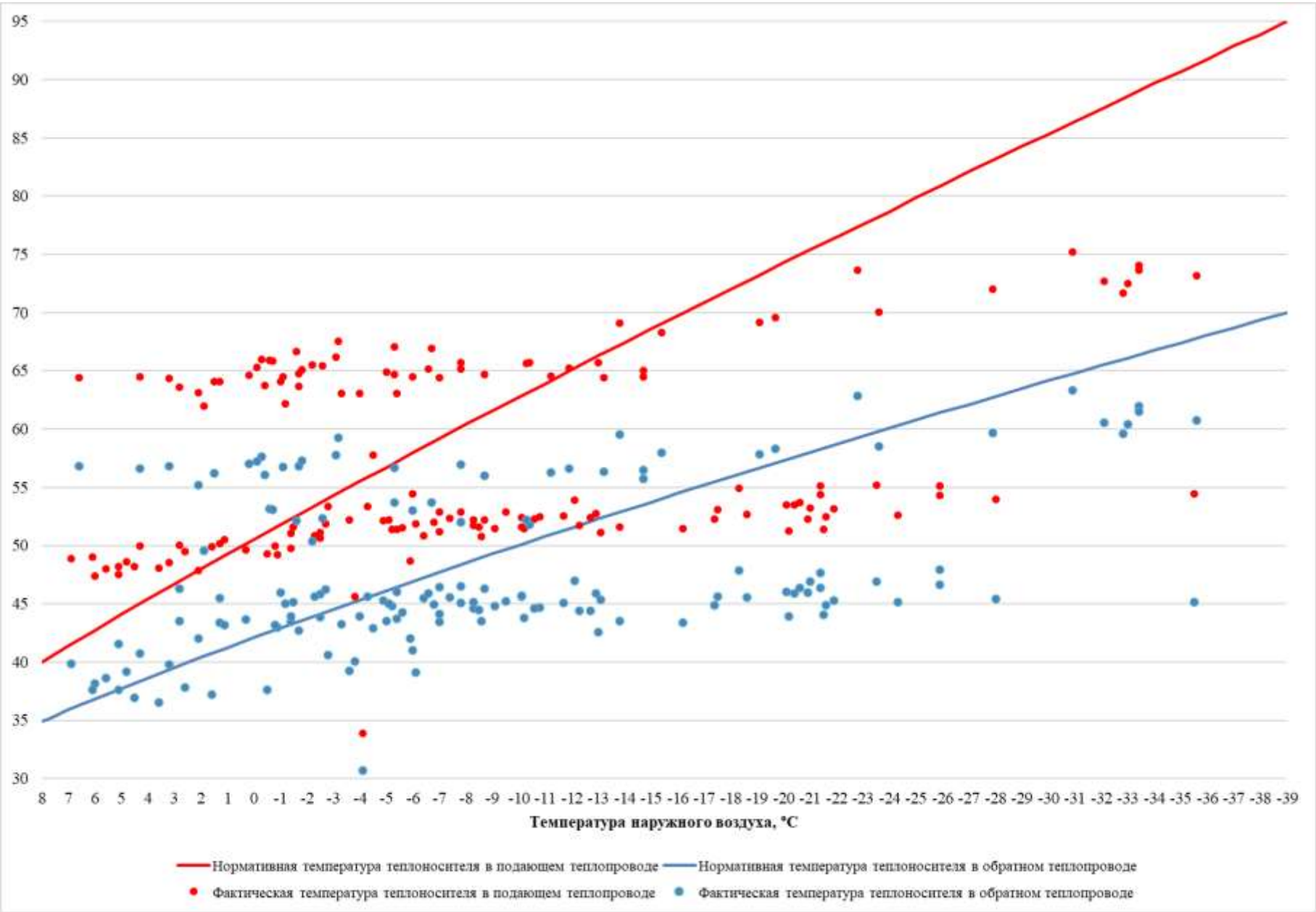
Рисунок 3.39 – Сравнение утвержденного и фактического температурных графиков за 2023 г. – Котельная школы №37
