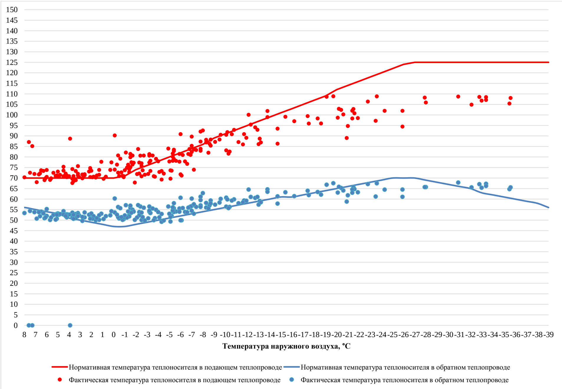
Рисунок 3.14 – Сравнение утвержденного и фактического температурных графиков за 2023 г. – ЦТЭЦ
