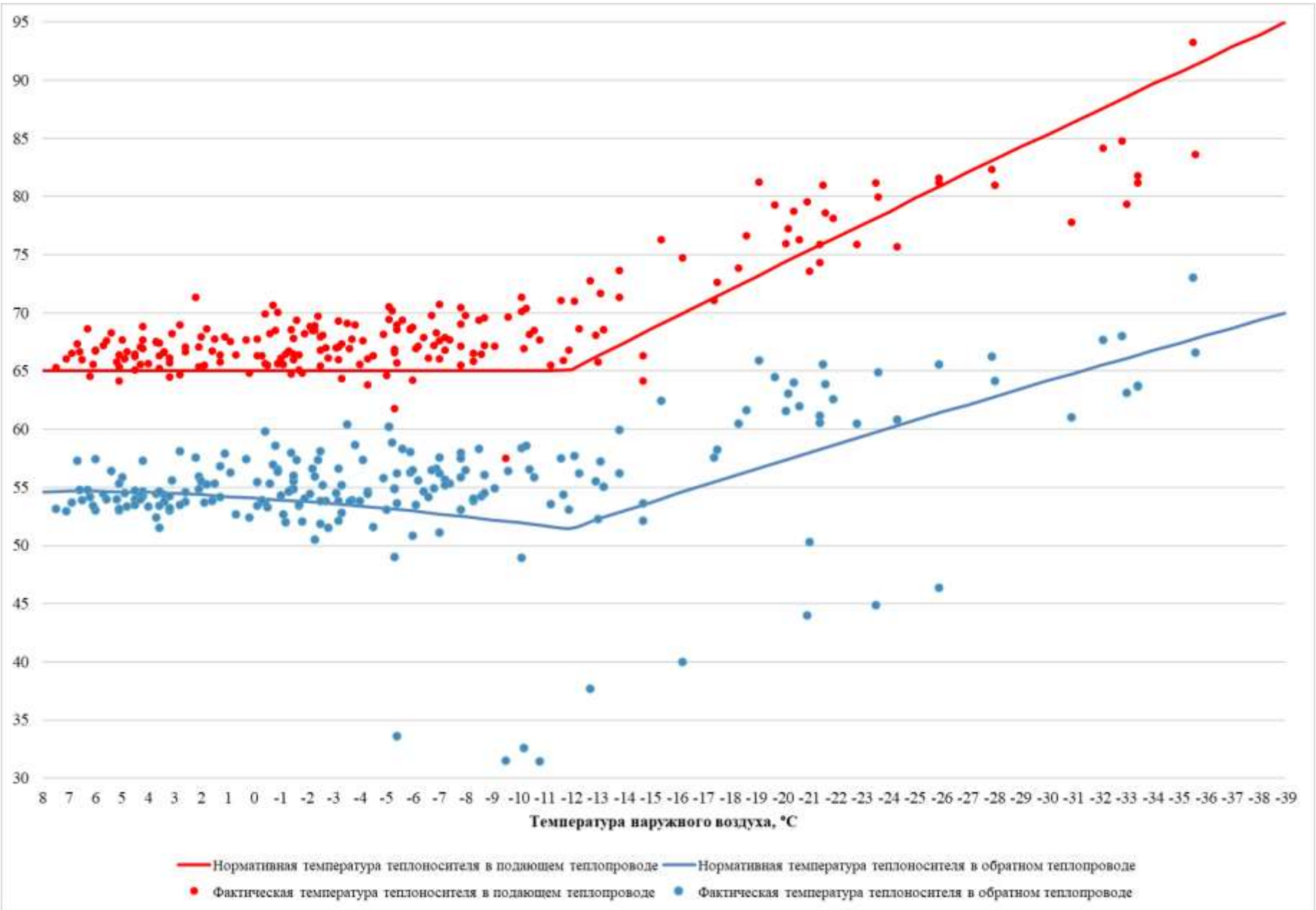
Рисунок 3.30 – Сравнение утвержденного и фактического температурных графиков за 2023 г. – Котельная №6
