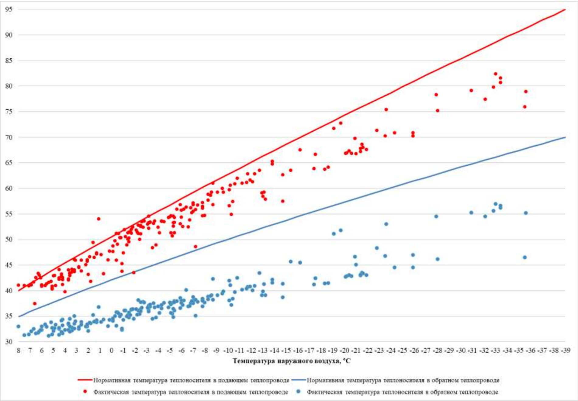
Рисунок 3.45 – Сравнение утвержденного и фактического температурных графиков за 2023 г. – Котельная «Кузнецкая крепость»
