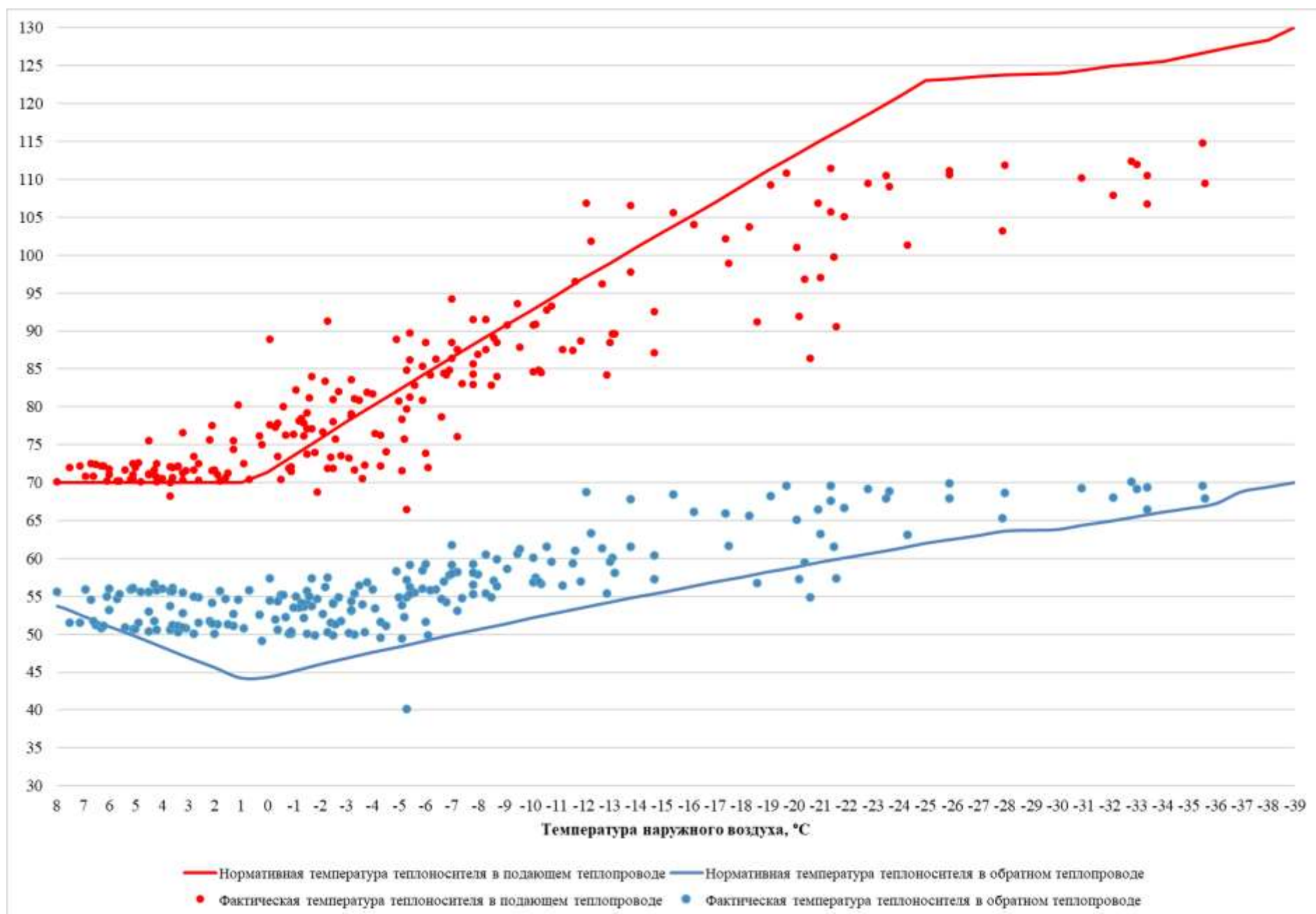
Рисунок 3.17 – Сравнение утвержденного и фактического температурных графиков за 2023 г. – Абашевская районная котельная
