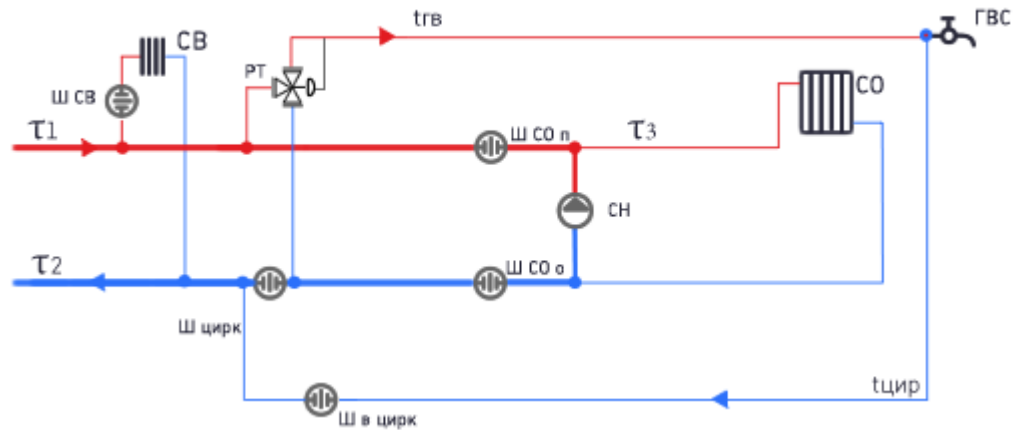
Рисунок 3.54 – Потребитель с открытым водоразбором на ГВС и насосным присоединением СО
