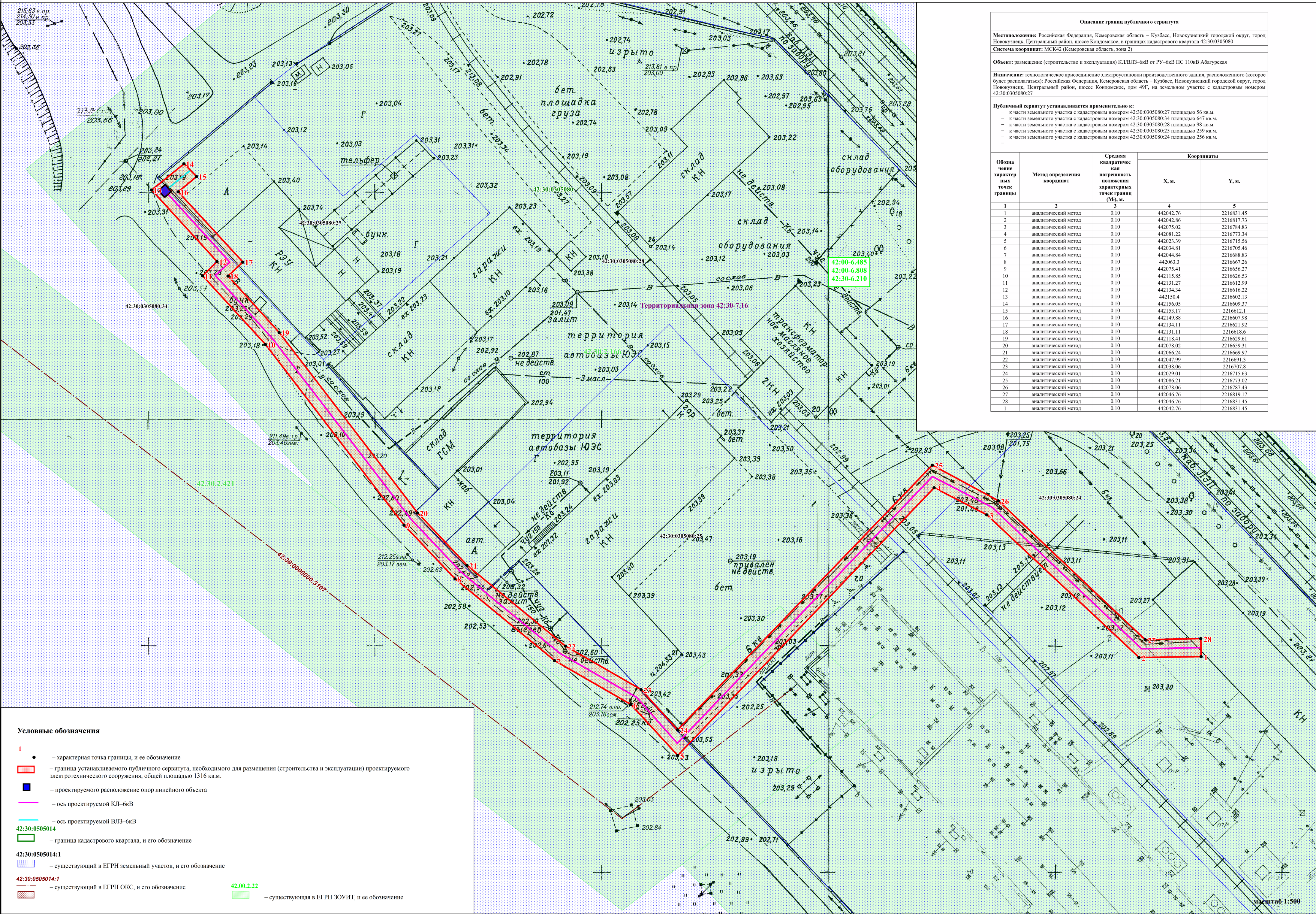
Схема расположения границ публичного сервитута
